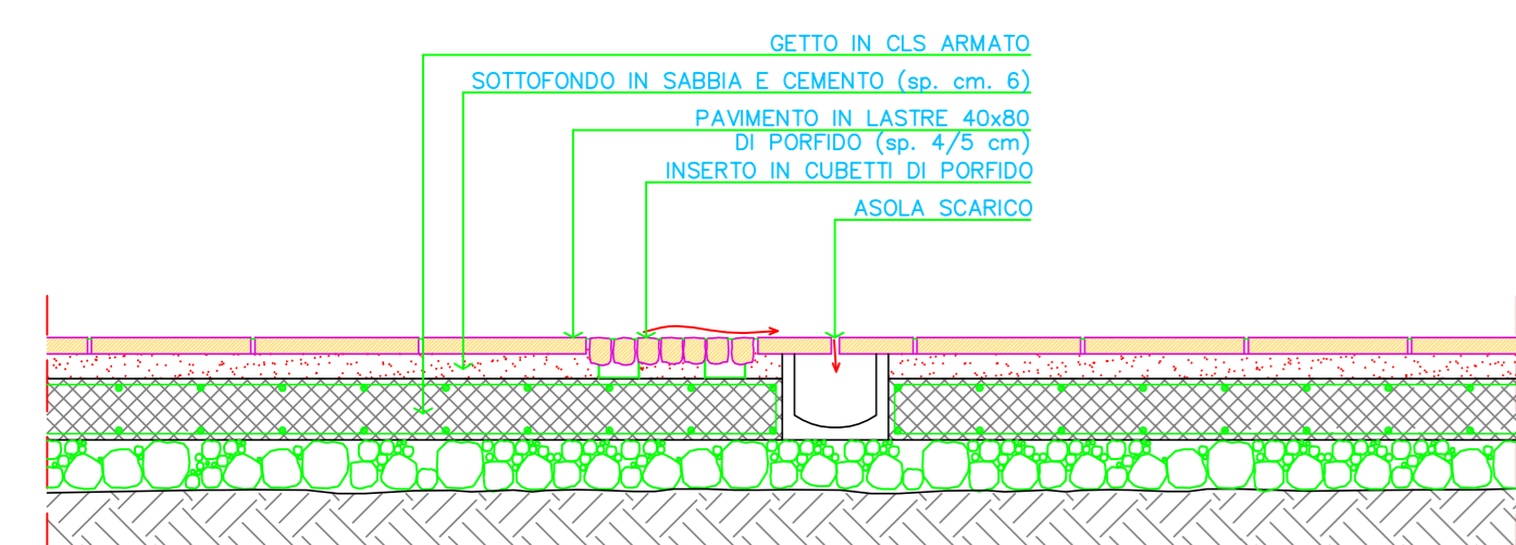
Sezione C-C
