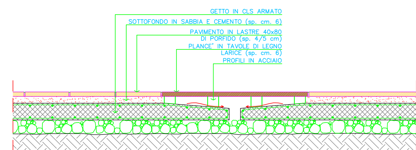
Sezione D-D
