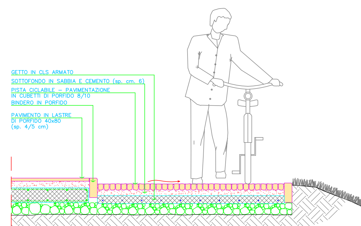
Sezione A-A pista ciclabile
