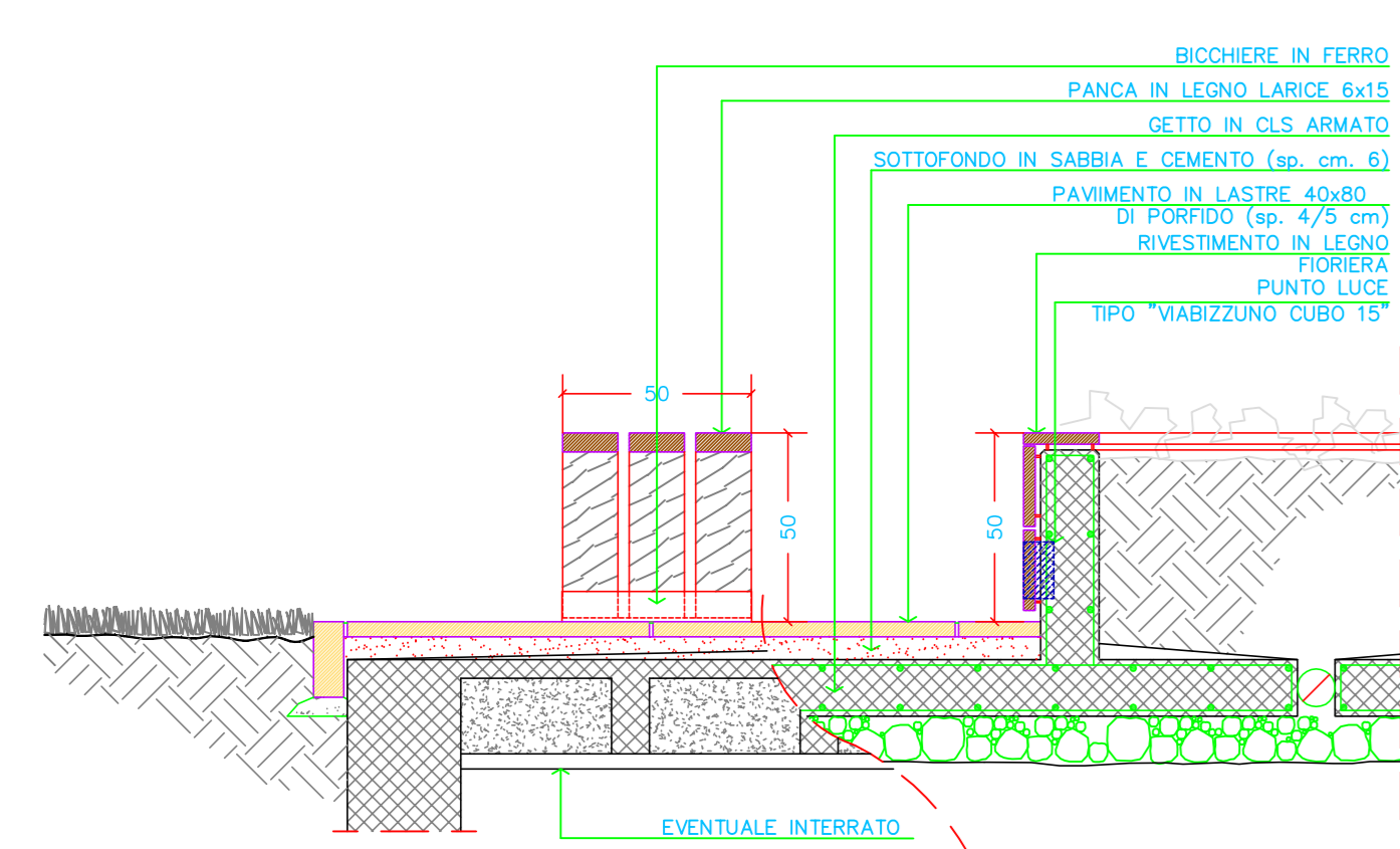
Sezione B-B fioriera/panca
